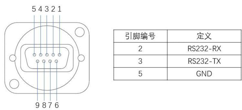
图 2.6 Q4 引脚说明图
